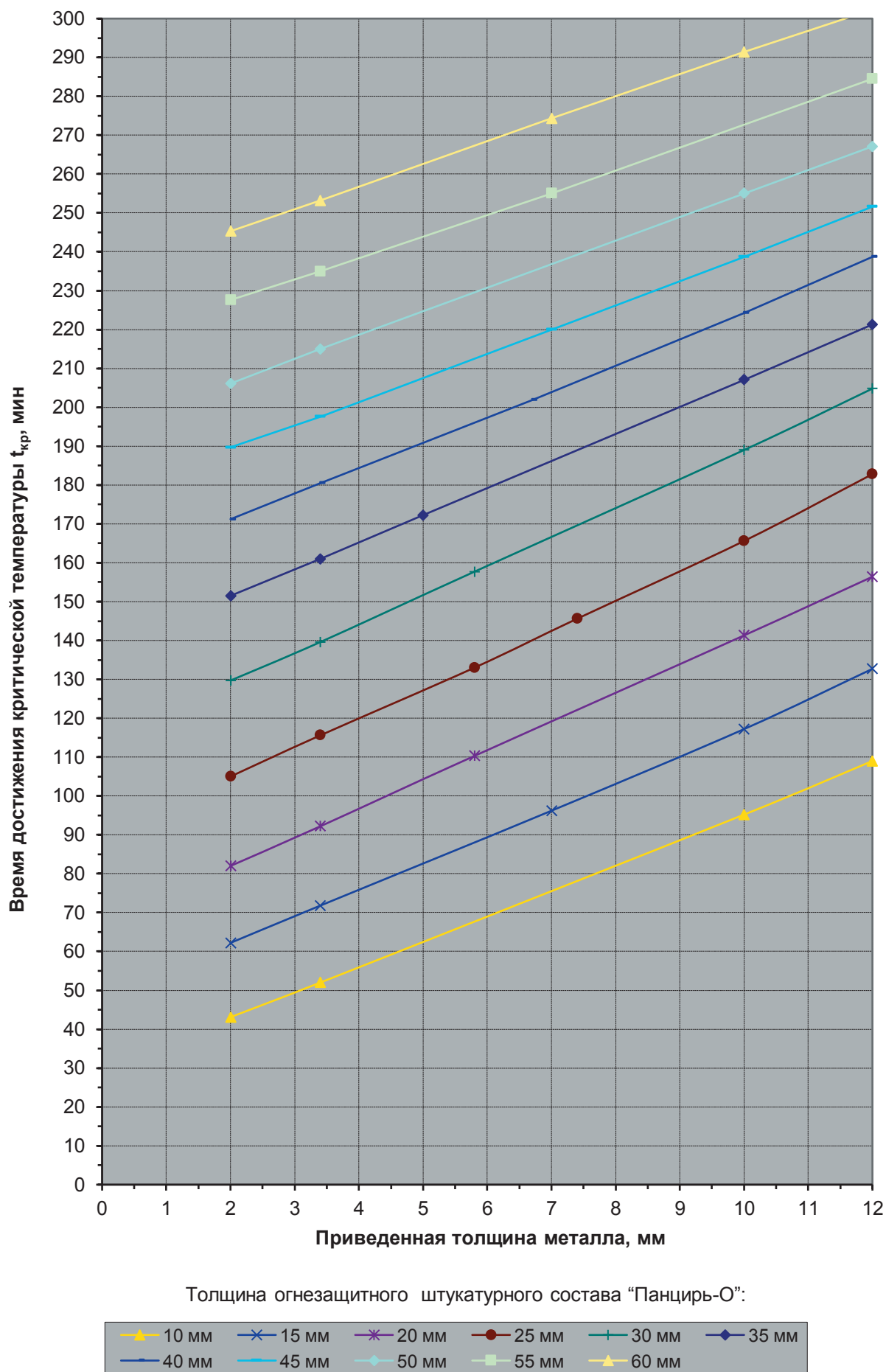
Рис. 21. Огнестойкость стальных конструкций с огнезащитным штукатурным составом "Панцирь-О" при t_{кр} = 550 \text{ }^\circ\text{C} .
