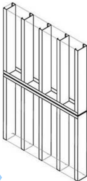
Рисунок 13 - Фрагмент КОС из каркасного модуля (МНК)
