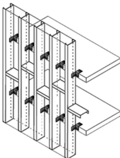
а) Стоечно-ригельный способ
