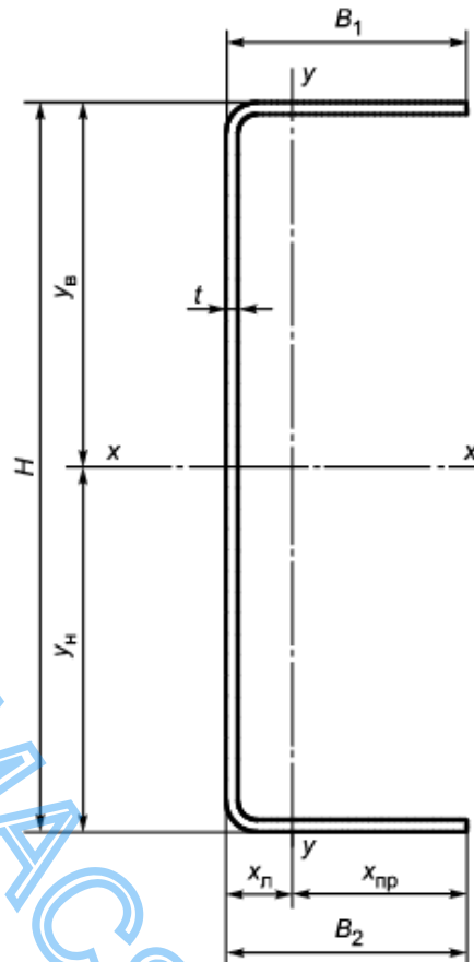
Рисунок Б.1 - Схема полного сечения швеллера
