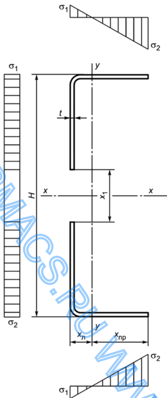
Рисунок Б.7 - Схема редуцированного сечения швеллера
