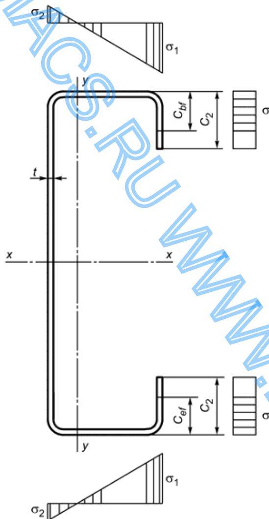
Рисунок Б.12 - Сечение С-образного профиля, изгибаемого относительно оси y-y , при сжатых отгибах полок
